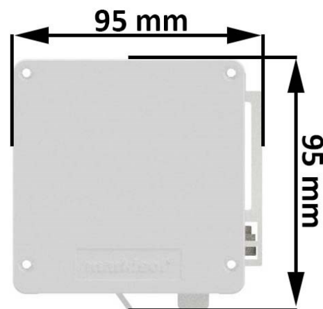
Montage på vägg
