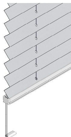
FJÄDERSPÄND SIDOSTRYNING MED LINA OCH PLASTFÄSTE
